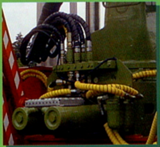
Les roulements à rouleaux de la base assurent à la grue une excellente sensibilité de mouvement.
